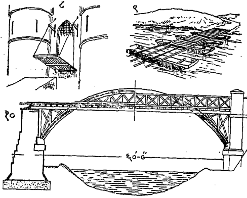
८. Draw bridge. : उचल. ९. Pontoon bridge. : पान्टून १०. Timber bridge. : फळ्यांचा (कमानदार).
